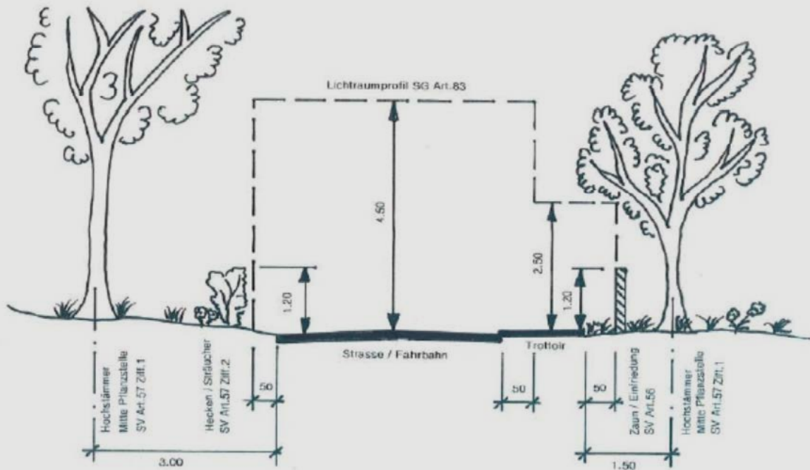
Skizze mit Lichtraumprofil mit den gesetzlichen Abständen an öffentlichen Strassen
